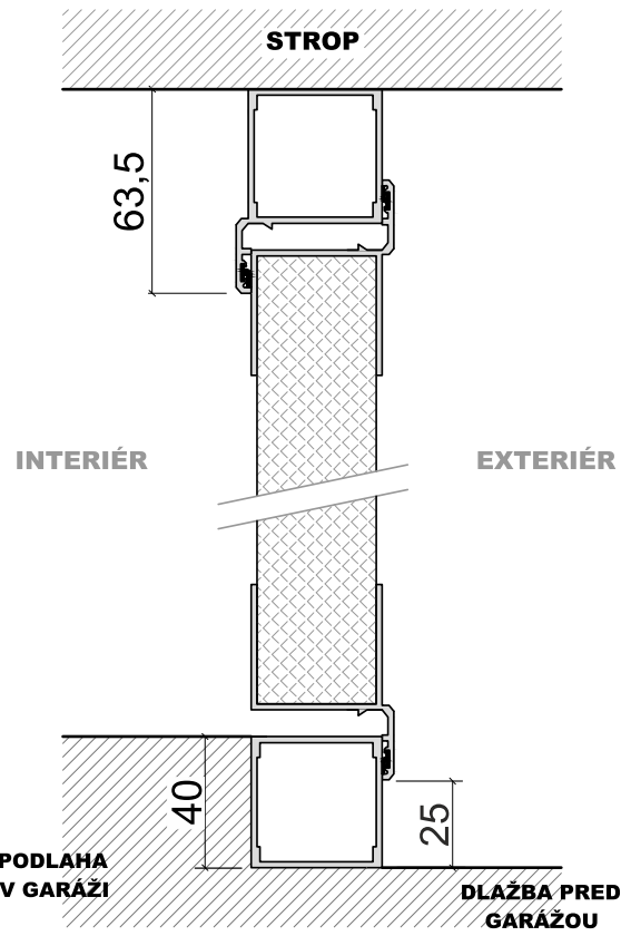
ZVISLÝ REZ KRÍDLOVOU BRÁNOU S HLINÍKOVÝM RÁMOM S PRAHOM ZAROVNO S PODLAHOU V INTERIÉRI A ZAROVNO S PODLAHOU V EXTERIÉRI
