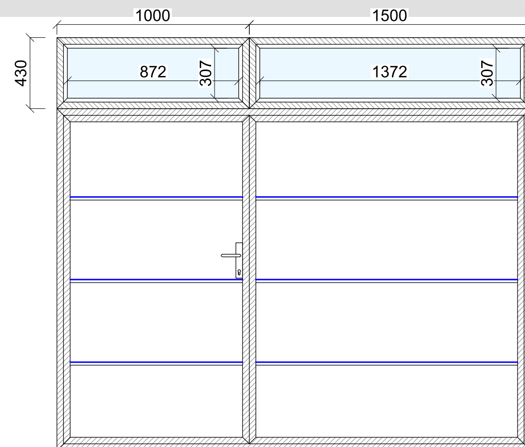
NESYMETRICKY DELENÁ DVOJKRÍDLOVÁ GARÁŽOVÁ BRÁNA S VODOROVNÝM NADSVETLÍKOM (pohľad zvonka)
