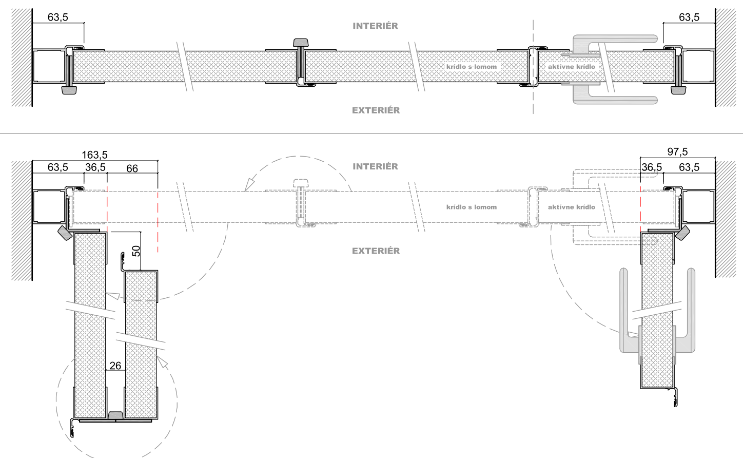
VODOROVNÝ REZ KRÍDLOVOU BRÁNOU S LOMOM S HLINÍKOVÝM RÁMOM OSADENIE BRÁNY DO OTVORU
