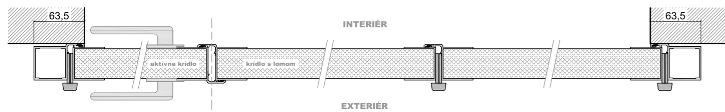
VODOROVNÝ REZ KRÍDLOVOU BRÁNOU S LOMOM S HLINÍKOVÝM RÁMOM OSADENIE BRÁNY PRED OTVOR
