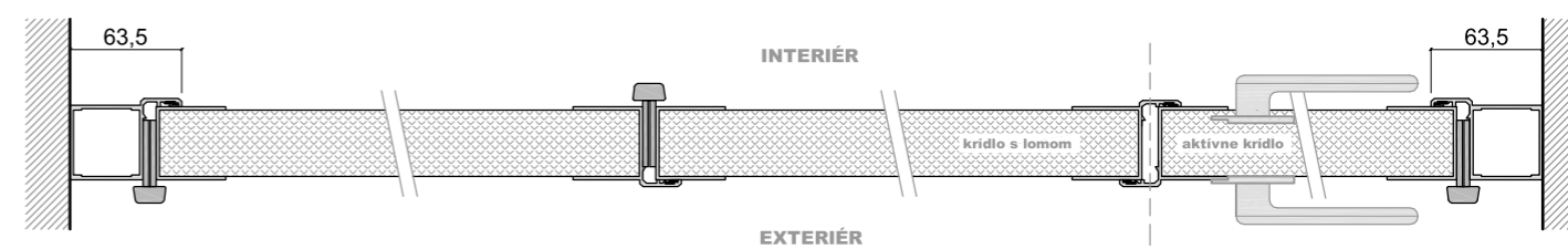
VODOROVNÝ REZ KRÍDLOVOU BRÁNOU S LOMOM S HLINÍKOVÝM RÁMOM OSADENIE BRÁNY DO OTVORU
