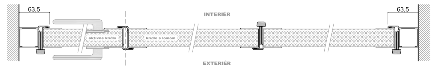
VODOROVNÝ REZ KRÍDLOVOU BRÁNOU S LOMOM S HLINÍKOVÝM RÁMOM OSADENIE BRÁNY DO OTVORU
